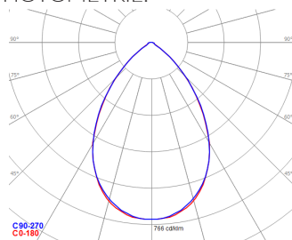
JUDO-3F_70_560W_4000K
